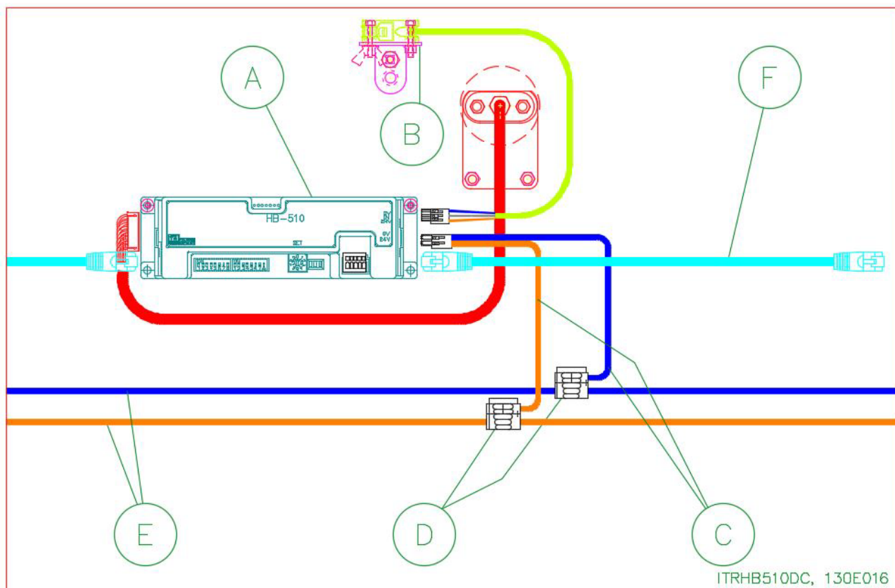
Figura 2: Tarjeta del controlador HB-510
